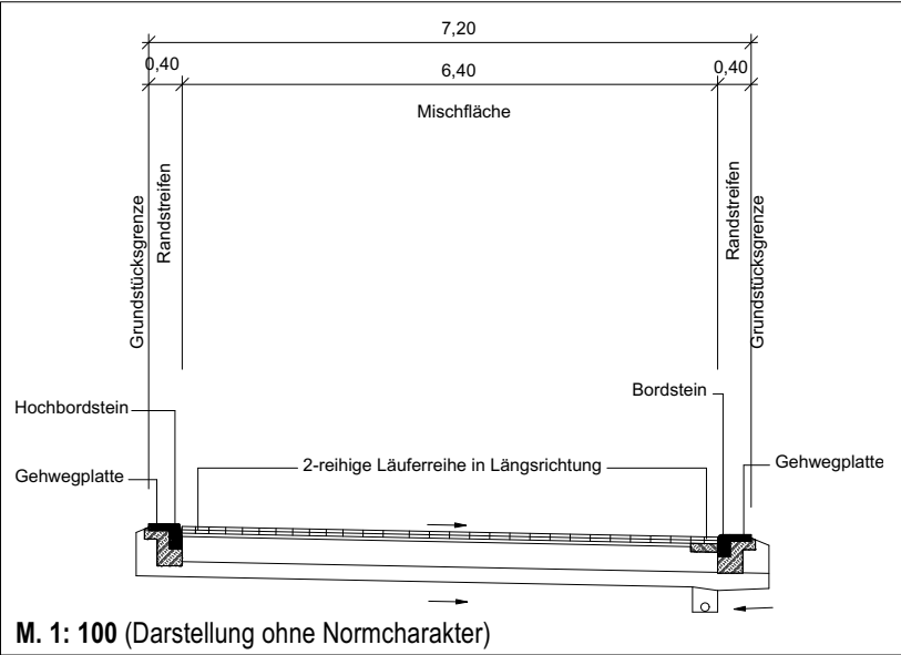
Straßenquerschnitt 1 Regelquerschnitt A-A' BvM-Bereich - ohne Parken
