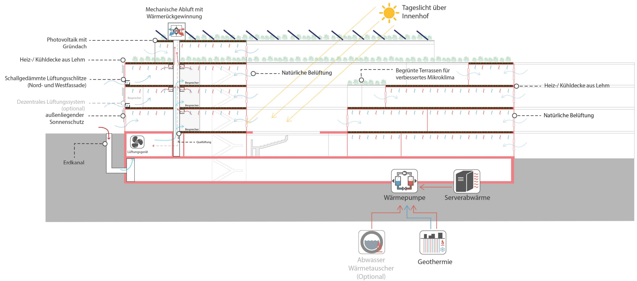
Energiekonzept (Stand Wettbewerb)
