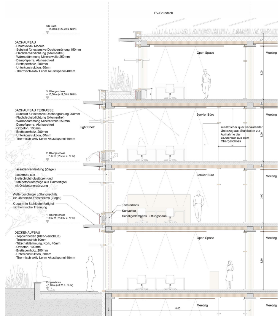
Fassadenschnitt (Stand Wettbewerb)
