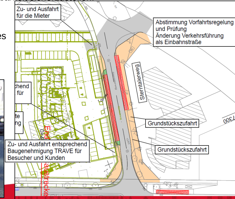
Abbildung: Lageplan Sterntaler Weg mit Planung TRAVE
