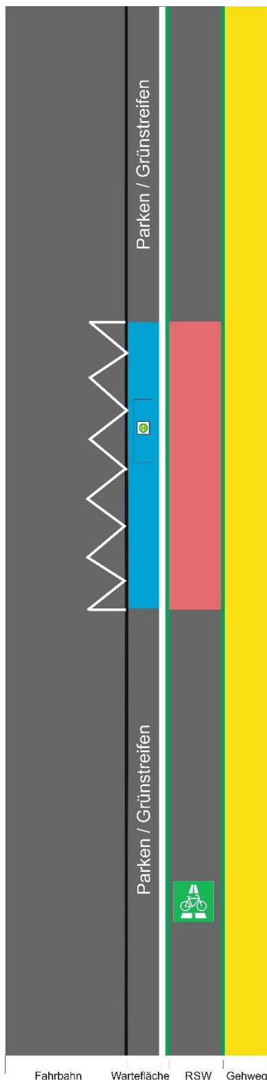
Abb. 6 RSW-Führung auf einem baulichen Radweg hinter der Bushaltestelle am Fahrbahnrand (Musterlösung 1)
