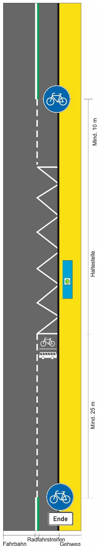
Abb. 8 RSW-Führung auf einem Radfahrstreifen, der für eine Bushaltestelle unterbrochen wird (Musterlösung 4)
