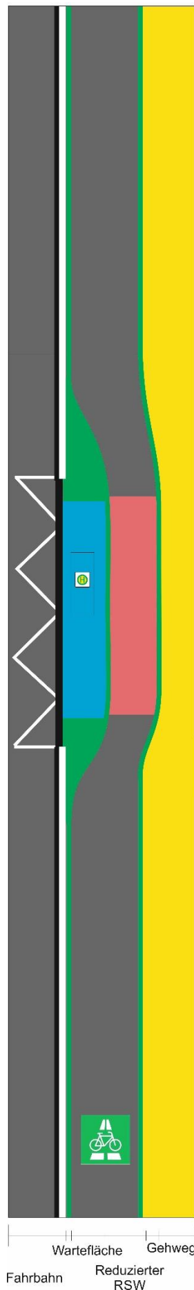
Abb. 7 RSW-Führung auf einem baulichen Radweg mit reduziertem Standard hinter der Bushaltestelle am Fahrbahnrand (Musterlösung 2)
