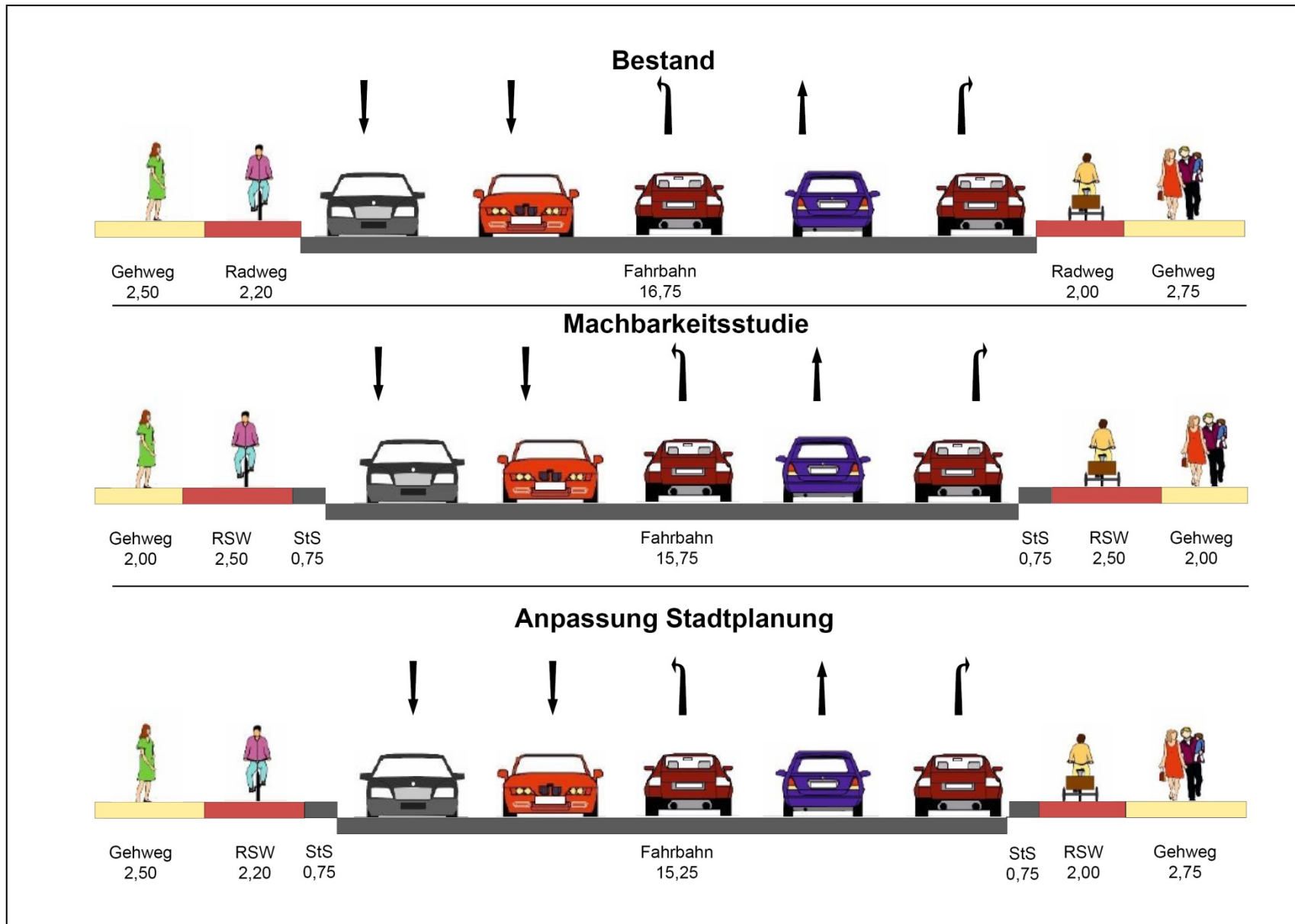
Abbildung 2: Querschnitt Teilstück a
