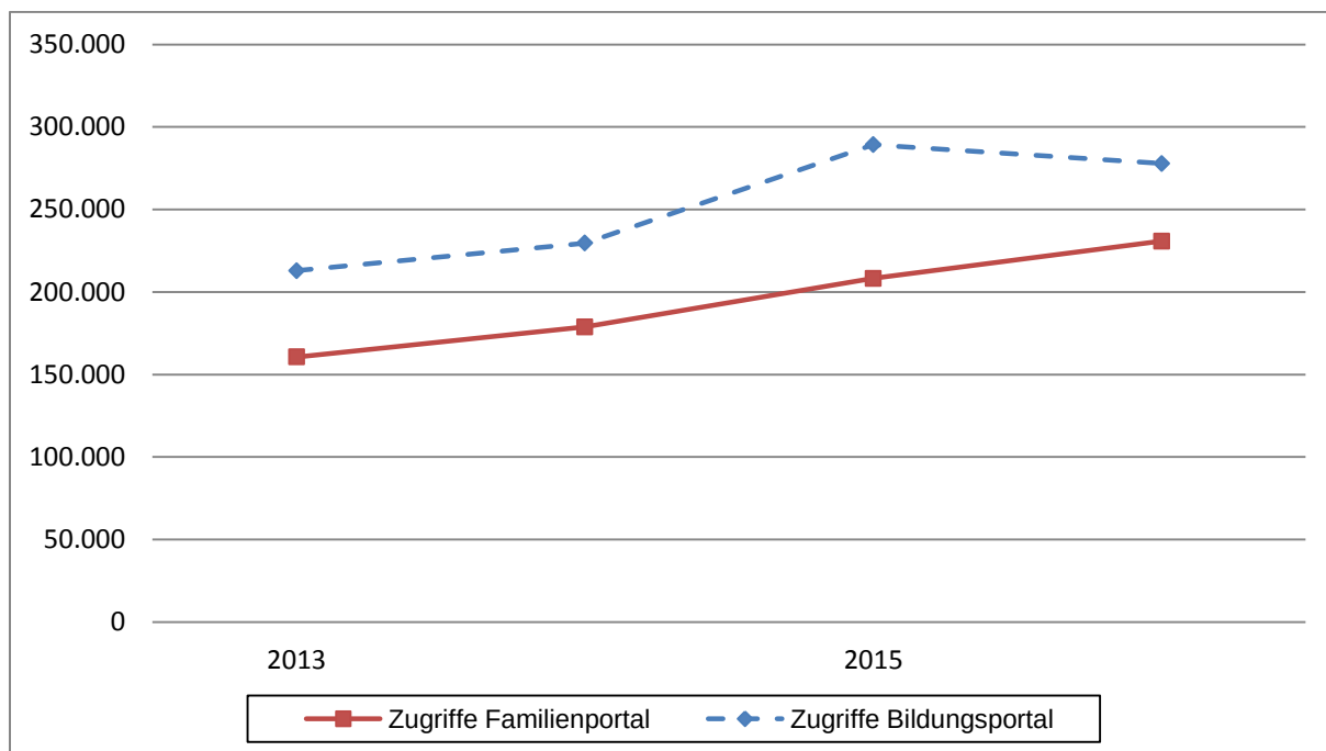
Abb. 8.1.1: Zugriffe Portale
