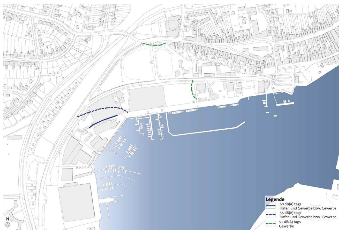
Abbildung 33: Lärmbelastung aus Gewerbe- und Hafenlärm bei freier Schallausbreitung - Tag
